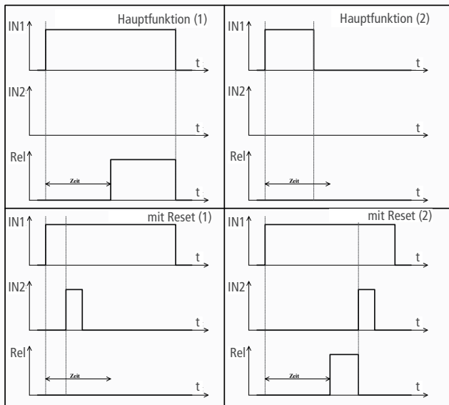
Funktion 1: Einschaltverzögerung mit Reset
