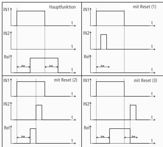
Funktion 3: Ein- und Ausschaltverzögerung mit Reset
