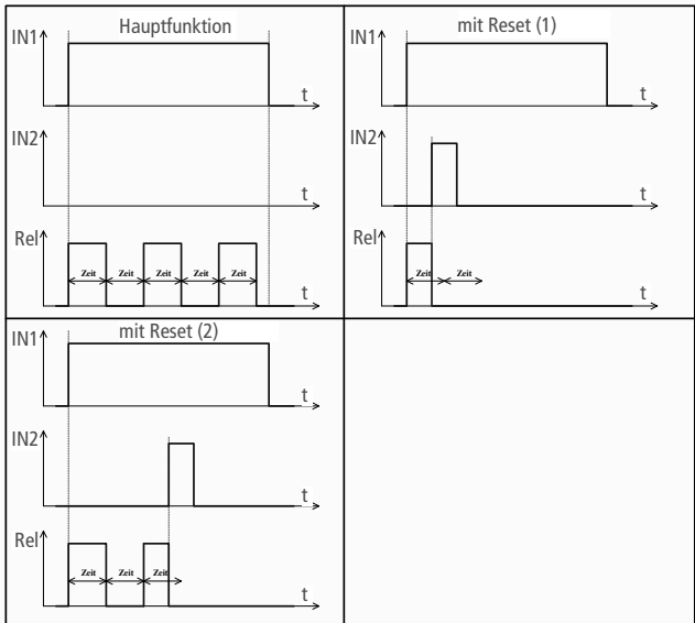
Funktion 8: Blinkschalter (Toggle) mit Reset
