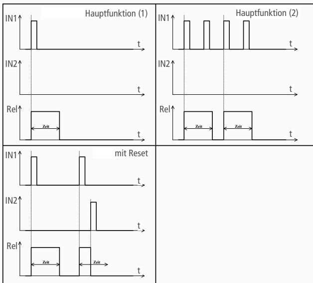
Funktion 4: Monoflop mit Reset
