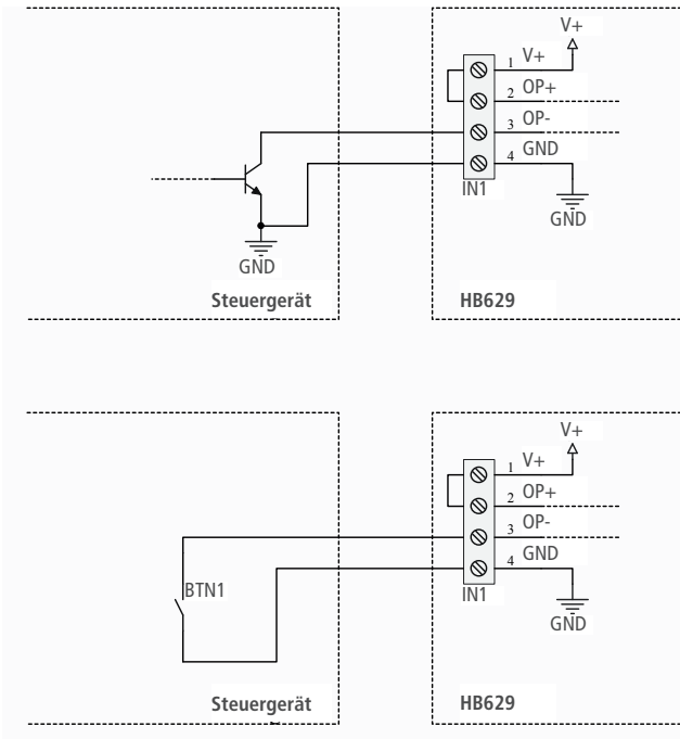
Beispiel N2: Ein Steueranschluss ohne galvanische Trennung
