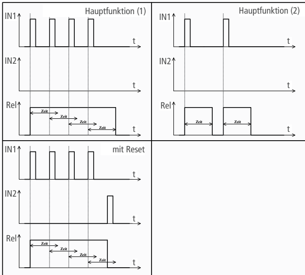
Funktion 5: Monoflop mit Restart und Reset
