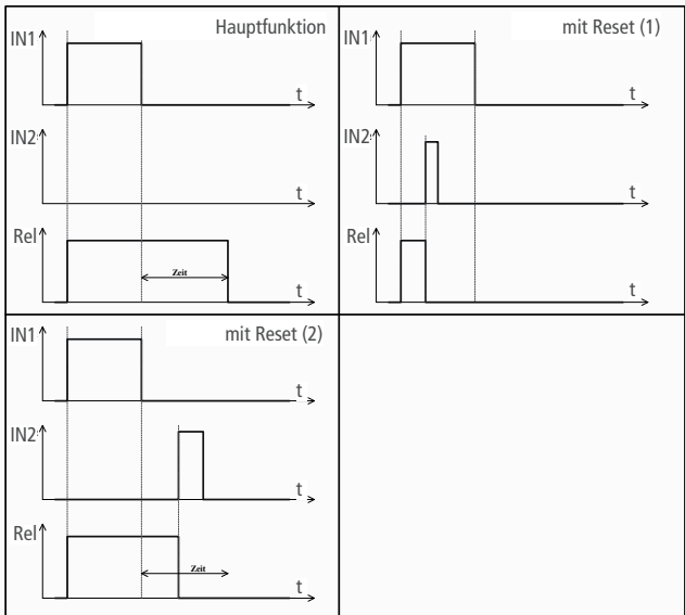
Funktion 2: Ausschaltverzögerung mit Reset
