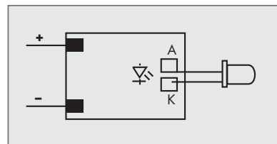
Anschluss-Skizze
